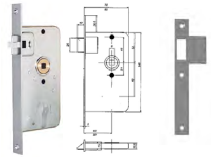
16.04F passage lock 16.05F passage lock 16.27F Passage
